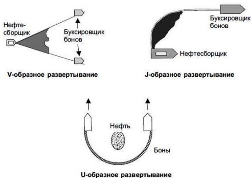
Рисунок 8.4 Схемы разворачивания оборудования в U-, J-, V-образных конфигурациях
