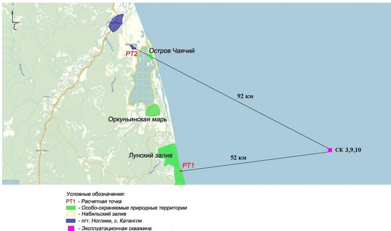
Рисунок 12.3 – Ситуационная карта-схема
